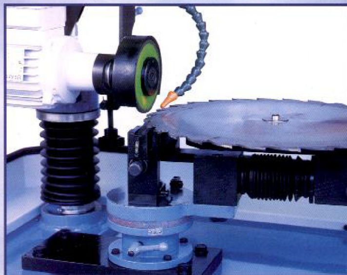
Regulation des angles de travail Einstellung des werkwinkel
