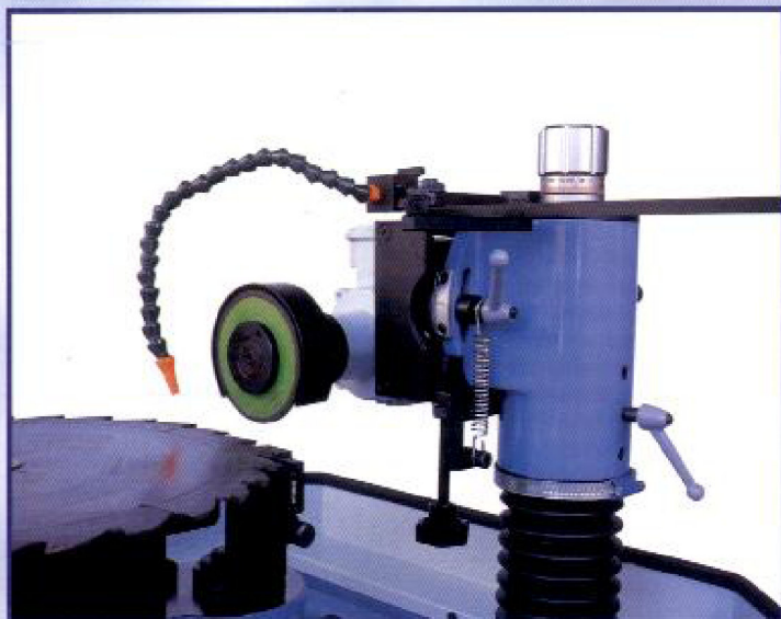
Regolazione angoli di lavoro Working angles set up
